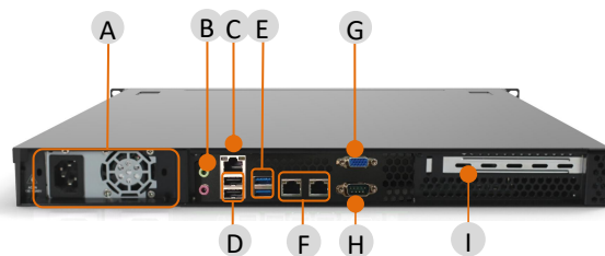
A: 电源 B: HD Audio C: IPMI D: USB 2.0 E: USB 3.0 F: LAN1/2 G: VGA H: COM I: PCI-E扩展槽
